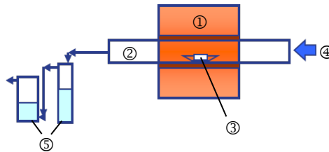
Abbildung 6: Prüfapparatur nach NF X 70-100 Figure 6: Test apparatus according to NF X 70-100
