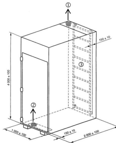
Abbildung 1: Kabelschacht nach EN 60332-3-10 Figure 1: Cable duct according to EN 60332-3-10
