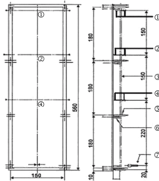
Abb.3: Prüfkörperhalter für die vertikale Brenngeschwindigkeit Fig.3: Specimen holder vor the vertical burning rate
